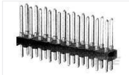
TE Part # 87215-1 08 MODII HDR DRST UNSHRD .100
