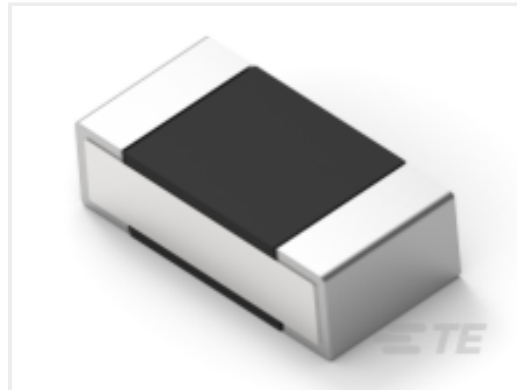
TE Part #5-2176310-5 RP 1E 0.1W 392R 0.1% 25PPM 1K RL
