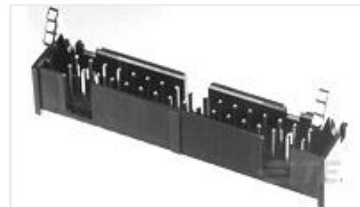
TE Part #1-1761606-1 IDC LOW PRO HDR 34P VERT LAT BLK
