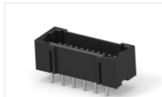
TE Part #4-292208-2 MINI CT D/R DIP 22P BLACK
