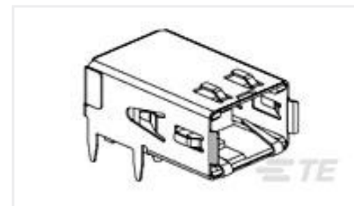
TE Part #1761072-3 RECPT,HSSDC2,FIBRE,TRAY PKG
