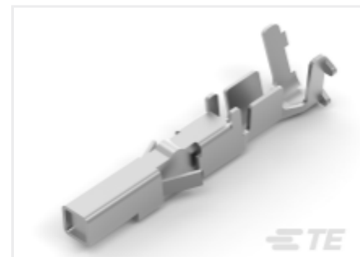
TE Part #2825213-1 VAL-U-LOK SKT HCS SN 22-18 LP
