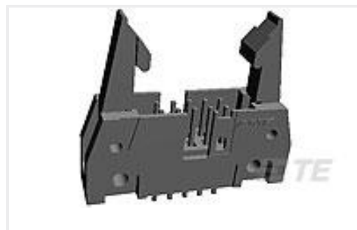
TE Part #5499160-1 A/L UNIV HDR 10P VERT SHT LAT
