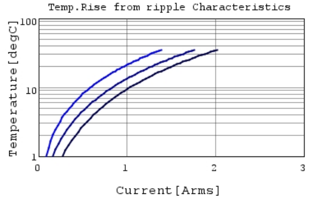
GRM155R61H224KE01 Temp.rise — 300kHz
