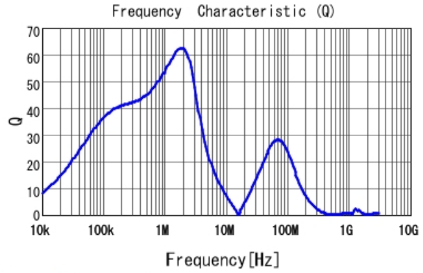
#B952AS-H-220M=P3 Q
