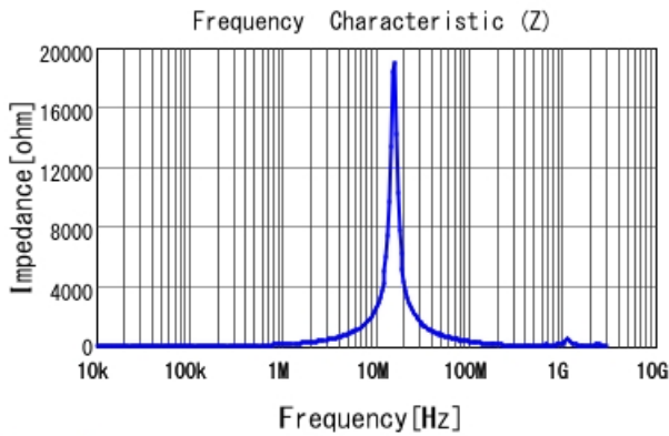
#B952AS-H-220M=P3 |Z|
