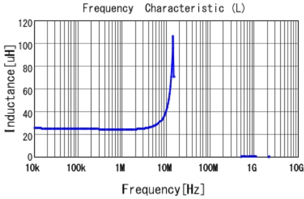
#B952AS-H-220M=P3 L
