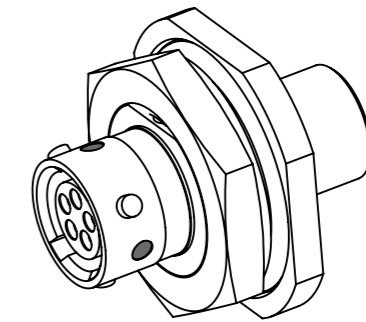
SCALE 2:1
