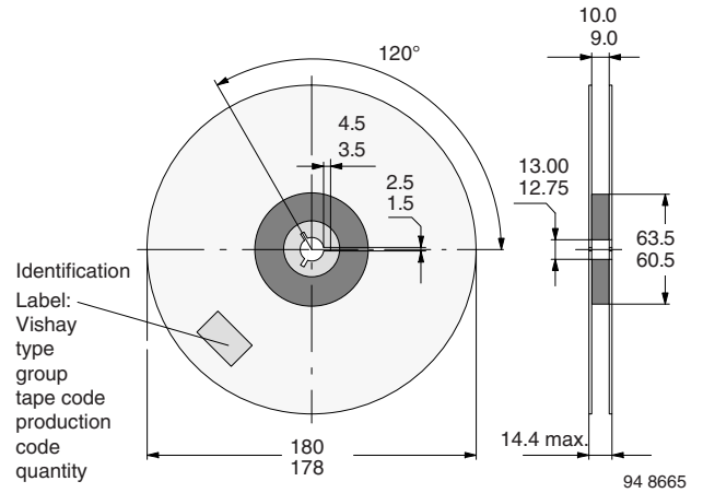
Fig. 24 - Reel Dimensions - GS08
