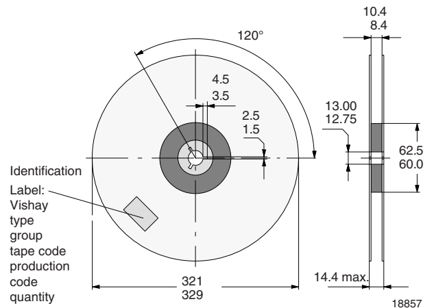
Fig. 25 - Reel Dimensions - GS18
