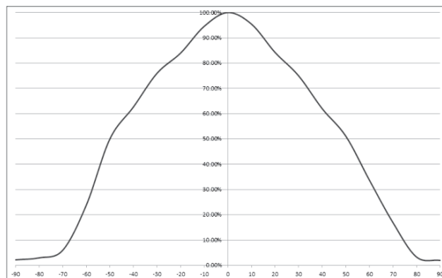
Fig. 7 - ALS View Angle
