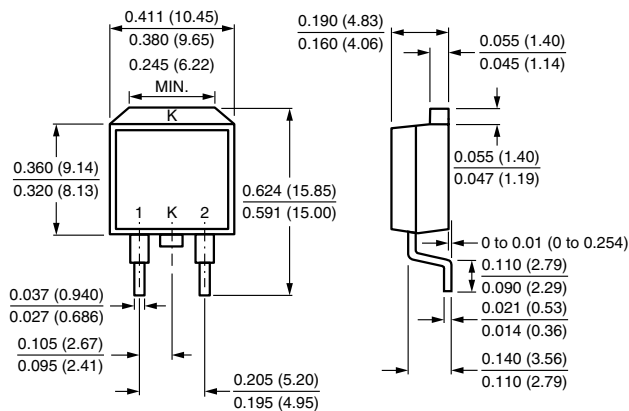
TO-263AB
