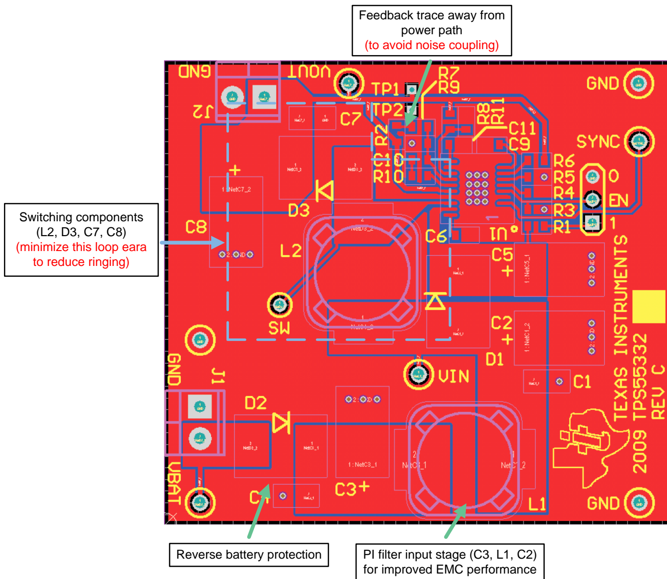
Figure 16. Top Layer
