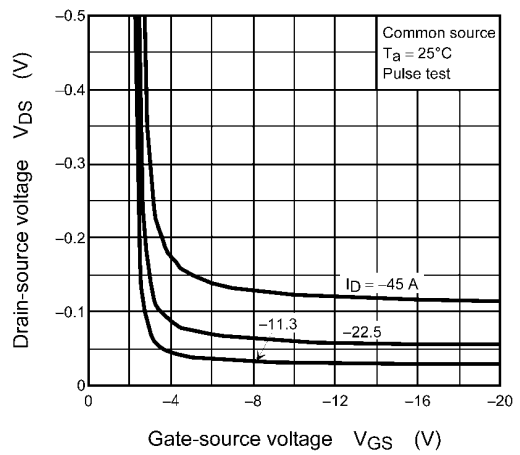
Fig. 8.4 V_{DS} - V_{GS}
