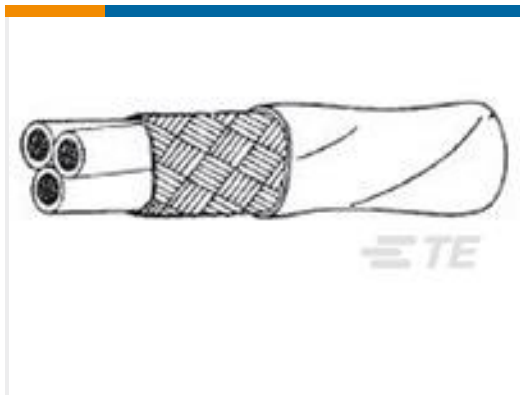
TE Part #316020-000 55A1131-24-2/4/6-9
