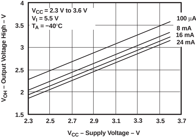
Figure 4. V_{OH} Values
