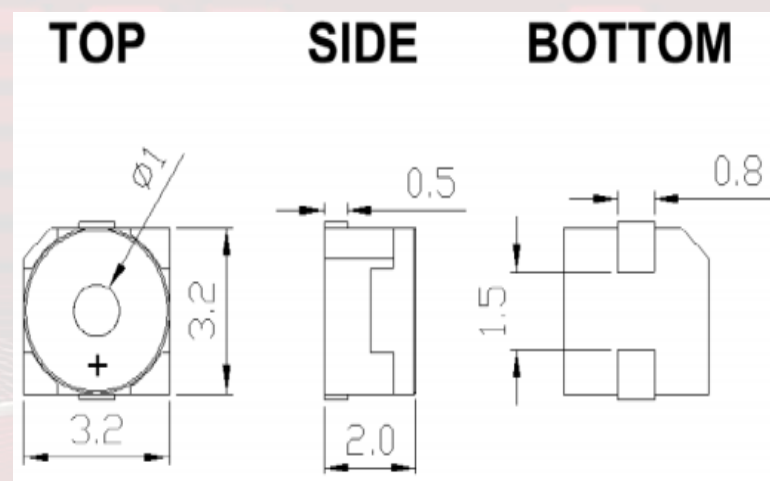
Dimensions
