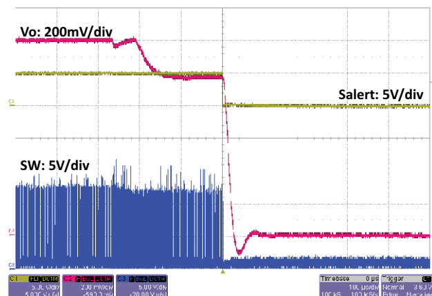
Fig. 33 - SiC451 UVP
