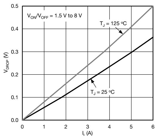
V_{DROP} vs. I_L at V_{IN} = 2.5\text{ V}
