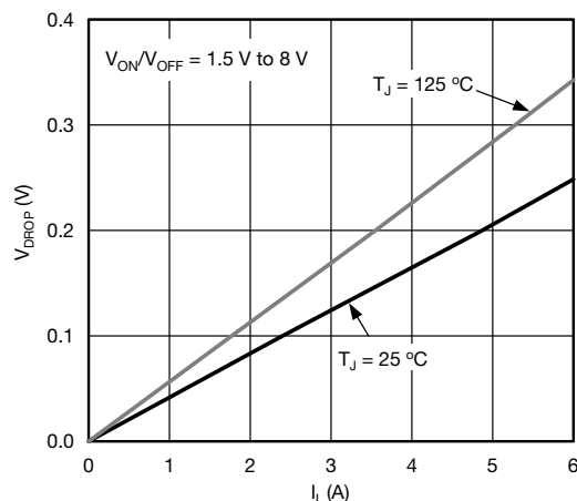
V_{DROP} vs. I_L at V_{IN} = 4.5\text{ V}
