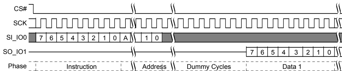
図 93. セキュリティ領域読み出しコマンド シーケンス
