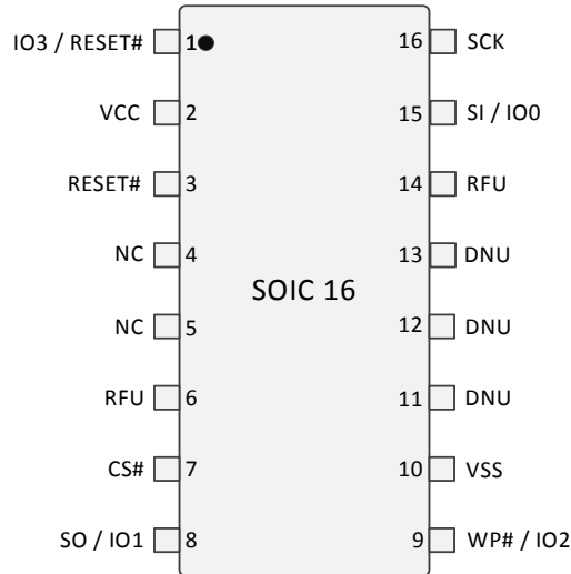
図 1. 16 リード SOIC パッケージ (SO3016)、上面図
