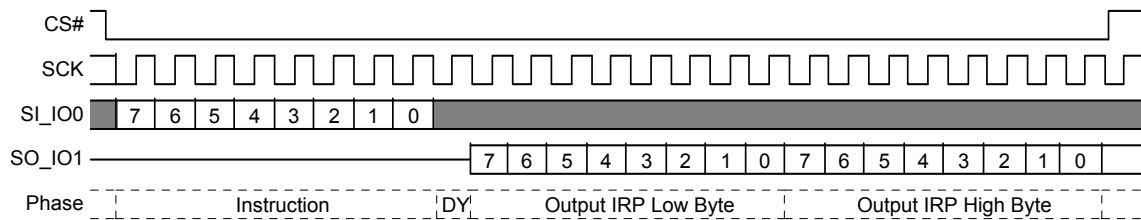
図 107. IRPRD コマンド シーケンス
