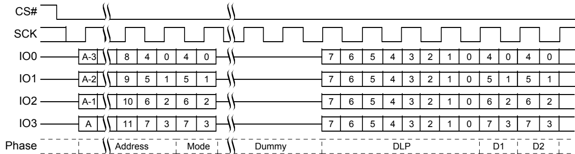
図 76. DDR クアッド I/O 連続読み出しの後続アクセス
