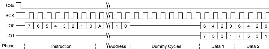
図 67. デュアル出力読み出しコマンド シーケンス
