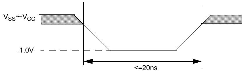
図 129. 最大負オーバーシュート波形
