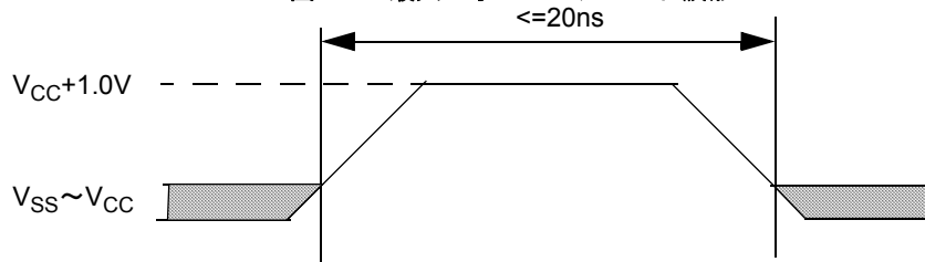
図 130. 最大正オーバーシュート波形
