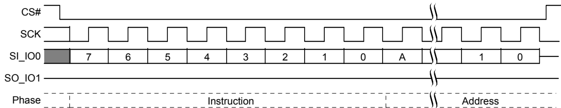
図 97. IBL コマンド シーケンス
