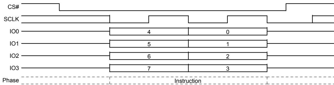
図 90. 消去/プログラム一時停止コマンドに続く命令コマンド シーケンス
