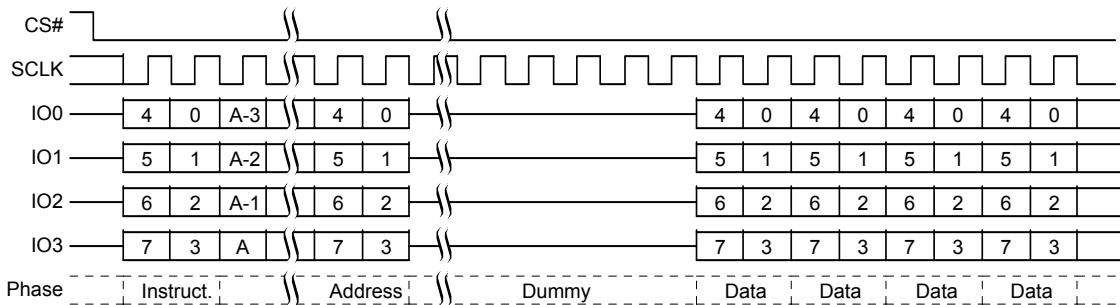
図 60. 任意レジスタ読み出しコマンド シーケンス - QPI モード
