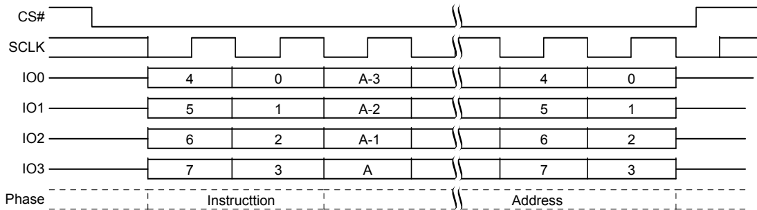
図 100. IBUL コマンド シーケンス - QPI モード
