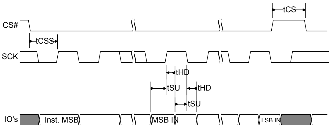
図 147. SPI DDR 入カタイミング
