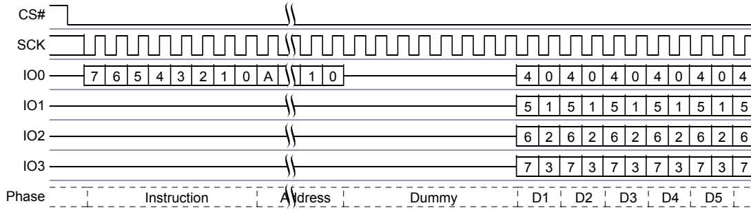
図 68. クアッド出力読み出しコマンド シーケンス
