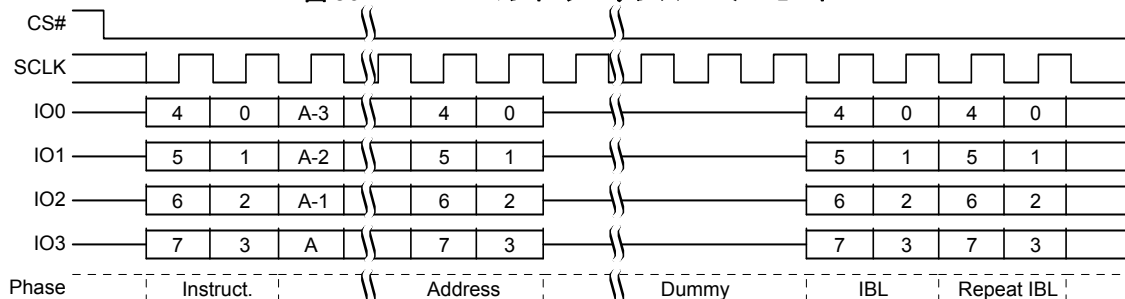
図 96. IBLRD コマンド シーケンス - QPI モード
