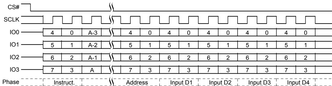
図 78. ページ プログラム (PP 02h または 4PP 12h) コマンド シーケンス - QPI モード
