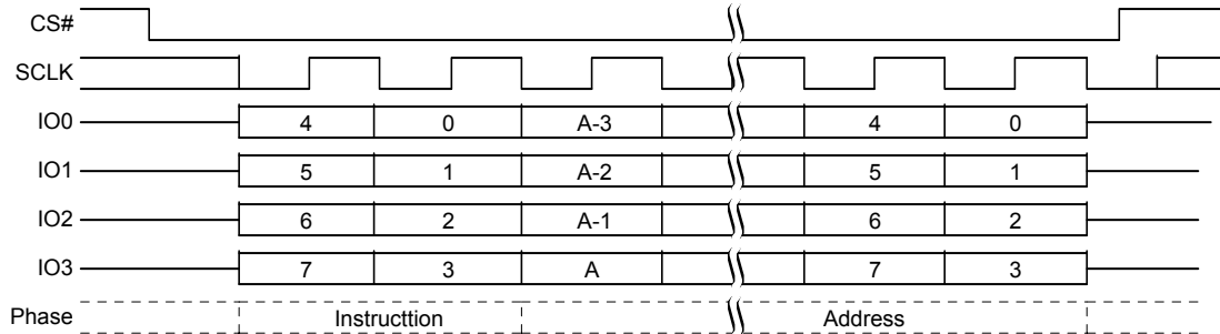
図 83. ハーフ ブロック 消去 (HBE 52h または 4HBE 53h) コマンド シーケンス - QPI モード
