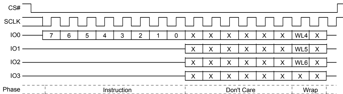
図 61. パースト長セット コマンド シーケンス – クアッド I/O モード
