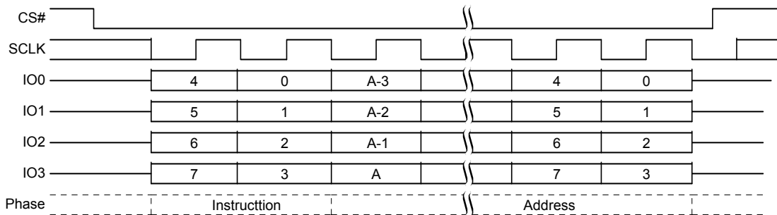
図 81. セクタ消去 (SE 20h または 4SE 21h) コマンド シーケンス – QPI モード
