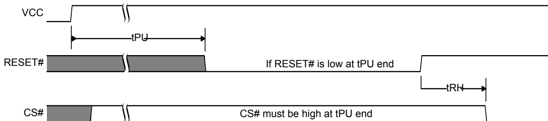
図 136. POR 終了時に RESET# LOW
