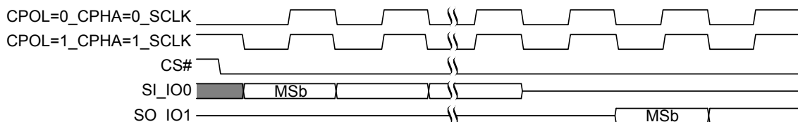
図 11. 対応の SPI SDR モード
