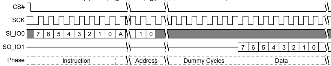
図 59. 任意レジスタ読み出しコマンド シーケンス
