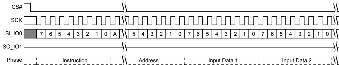
図 77. ページ プログラム (PP 02h または 4PP 12h) コマンド シーケンス
