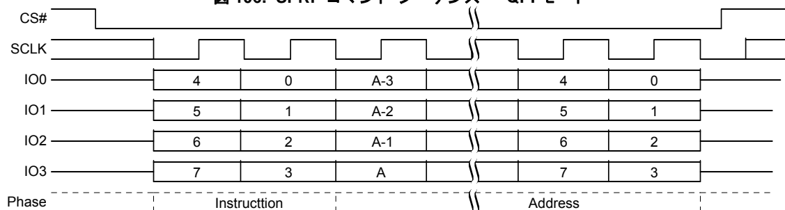
図 106. SPRP コマンド シーケンス - QPI モード
