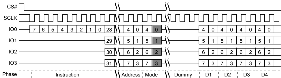
図 20. クアッド I/O コマンド
