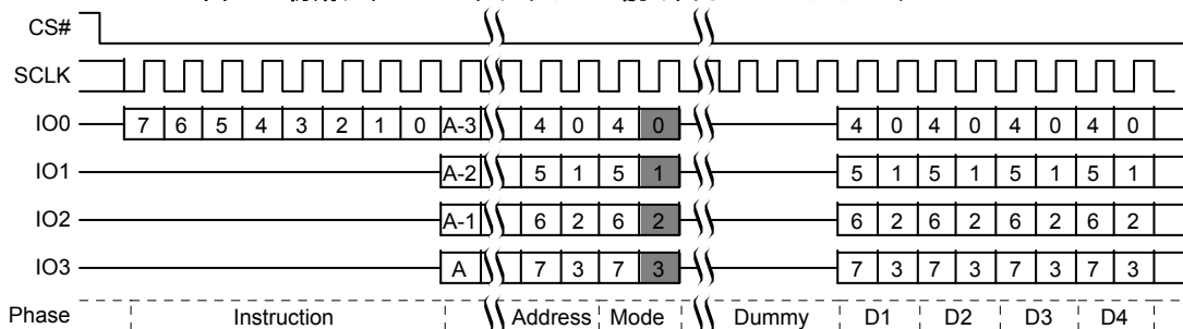
図 71. 初期アクセスのクアッド I/O 読み出しコマンド シーケンス
