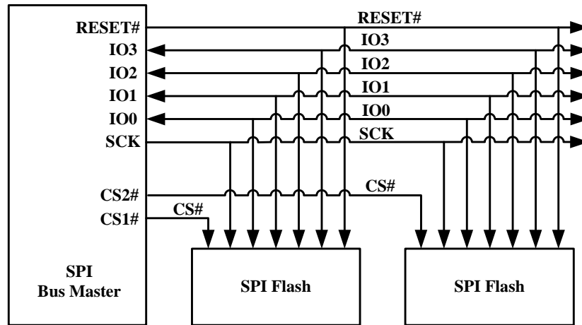
図 9. SPIバス上のバス マスターおよびメモリ デバイス – クアッド ビット データ パス – 個別 RESET#
