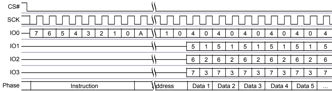
図 79. クアッド ページ プログラム コマンド シーケンス
