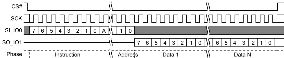
図 65. 読み出しコマンド シーケンス
