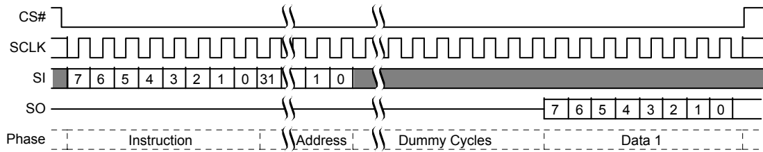
図 16. レイテンシ付きのシングルビット幅の I/O コマンド
