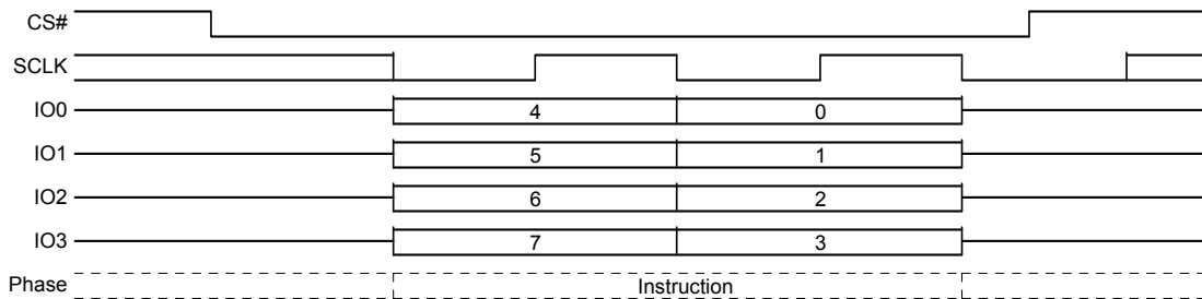
図 48. ステータスレジスタクリア (CLSR) コマンド - QPI モード
