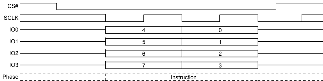
図 102. グローバル IBL ロック (GBL) コマンド シーケンス - QPI モード
