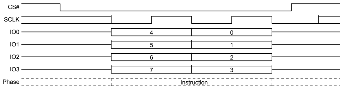
図 58. 4 バイト アドレス モード終了 – QPI モード
