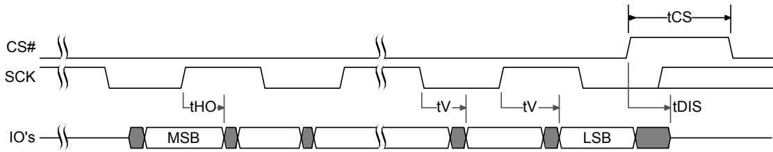
図 148. SPI DDR 出力タイミング
