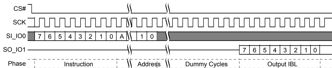
図 95. IBLRD コマンド シーケンス
