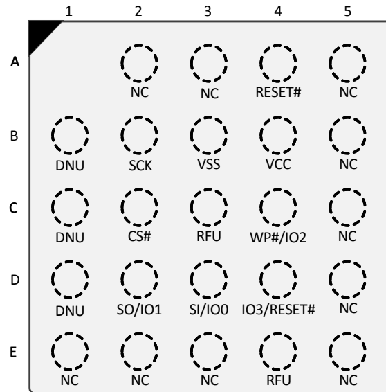
図 4. 24 ボール BGA、5x5 ボール フットプリント (FAB024)、上面図
