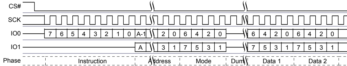
図 69. デュアル I/O 読み出しコマンド シーケンス
