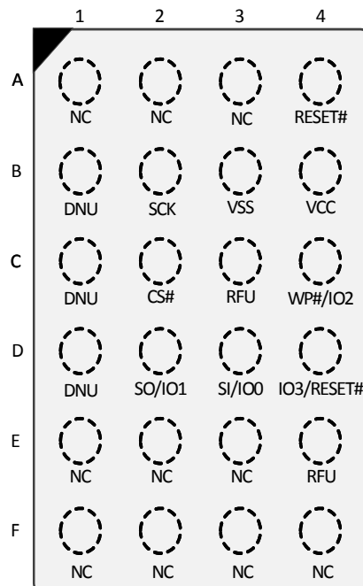
図 5. 24 ボール BGA、4x6 ボール フットプリント (FAC024)、上面図
