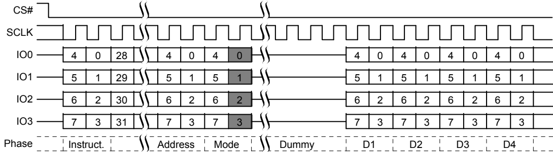
図 21. クアッド I/O 読み出しコマンド - QPI モード
