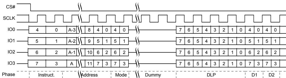
図 75. DDR クアッド I/O 読み出しの初期アクセス - QPI モード
