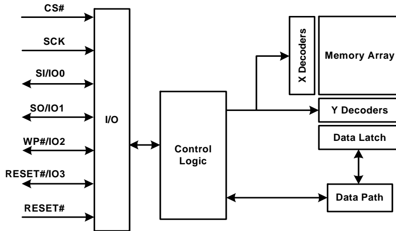
図 6. 論理ブロック図
