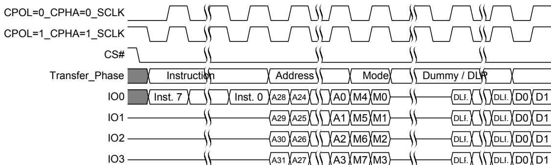
図 12. 対応の SPI DDR モード
