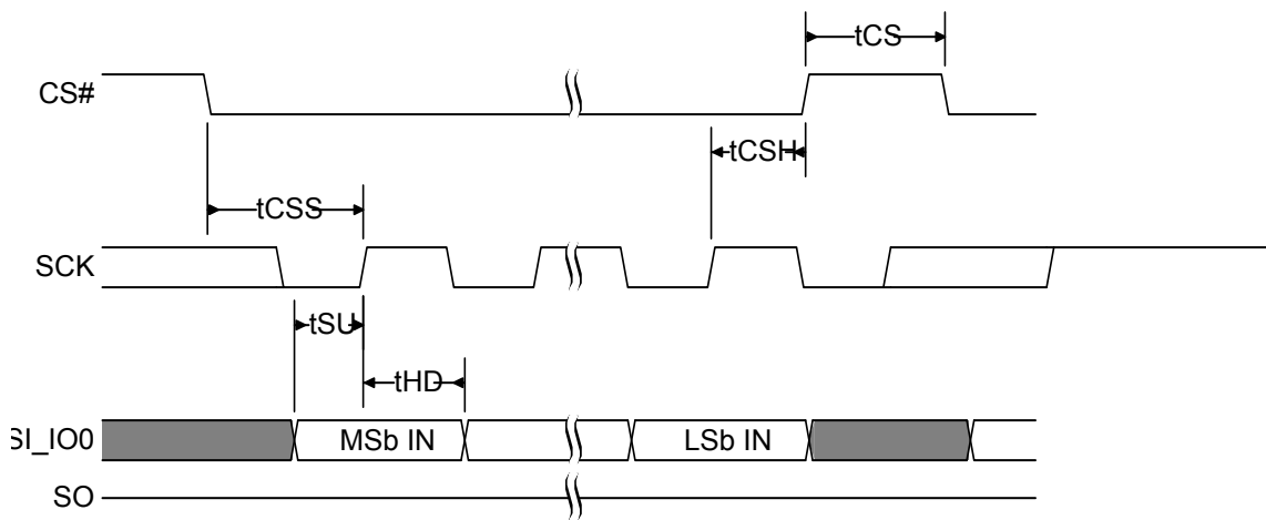
図 143. SPI シングル ビットの 入力 タイミング
