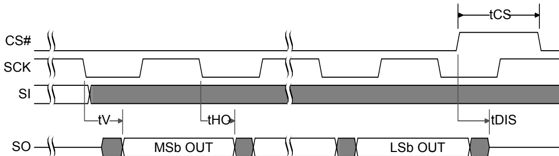
図 144. SPI シングル ビットの 出力 タイミング
