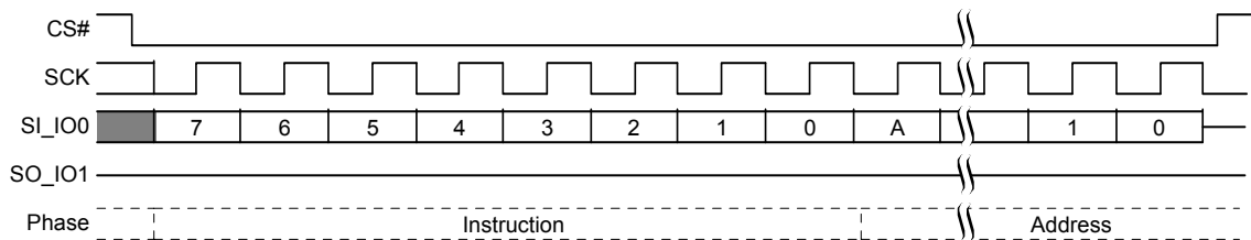
図 80. セクタ消去 (SE 20h または 4SE 21h) コマンド シーケンス
