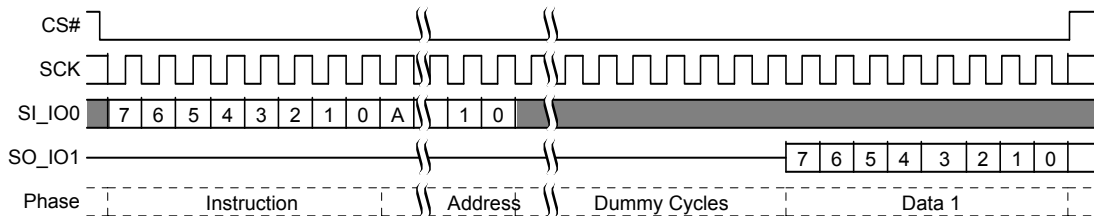
図 31. RSFDP コマンド シーケンス
