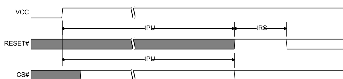
図 138. POR 後にハードウェアリセットが続く
