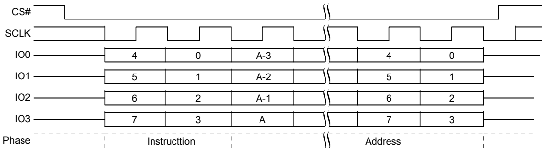
図 98. IBL コマンド シーケンス - QPI モード
