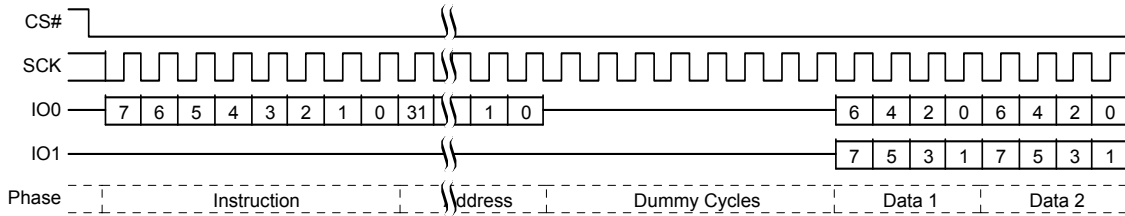
図 17. デュアル出力の読み出しコマンド
