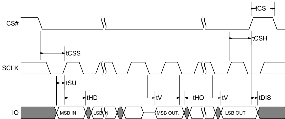
図 145. SDR MIO タイミング
