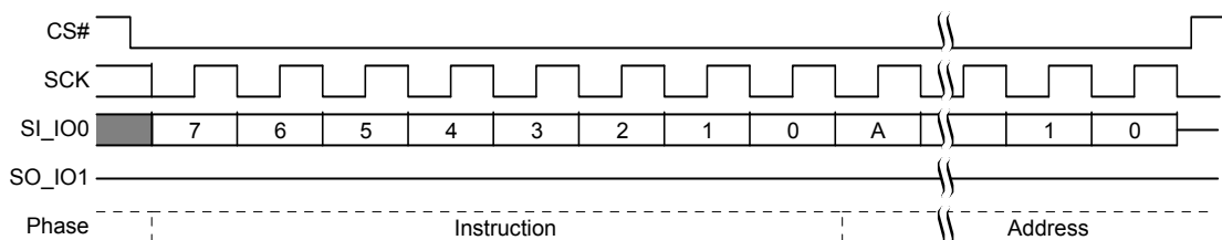
図 84. ブロック消去 (BE D8h または 4BE DCh) コマンド シーケンス
