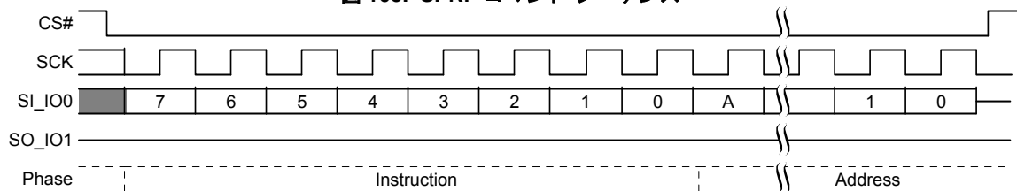
図 105. SPRP コマンド シーケンス
