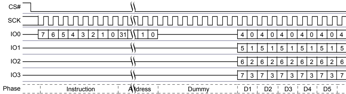
図 18. クアッド出力の読み出しコマンド
