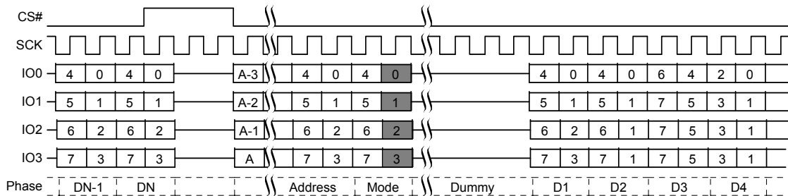
図 73. クアッド I/O 連続読み出しコマンド シーケンス
