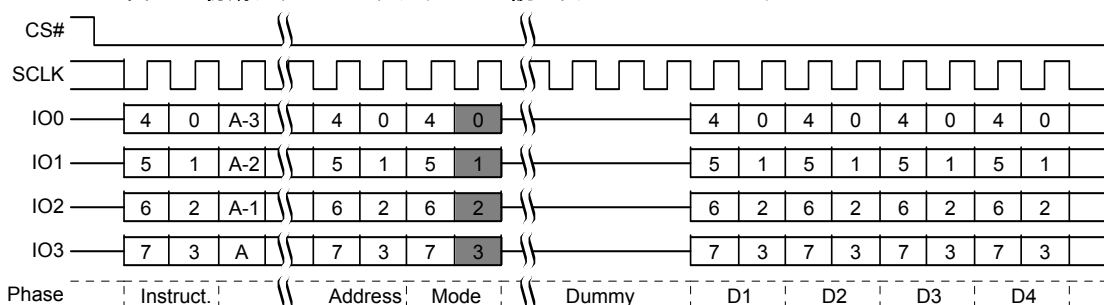
図 72. 初期アクセスのクアッド I/O 読み出しコマンド シーケンス - QPI モード
