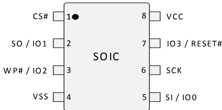
図 2. 8 ピン プラスチック小型パッケージ (SOIC8)
