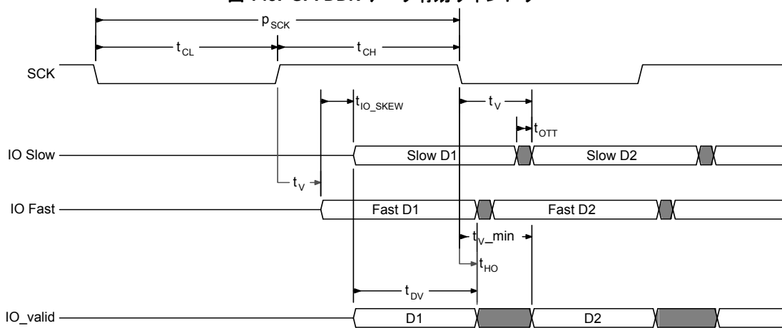
図 149. SPI DDR データ有効ウィンドウ
