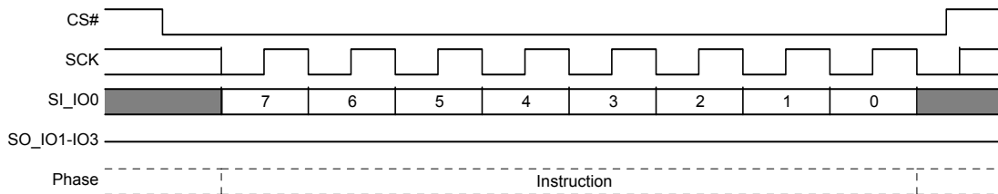
図 13. スタンドアロン命令コマンド
