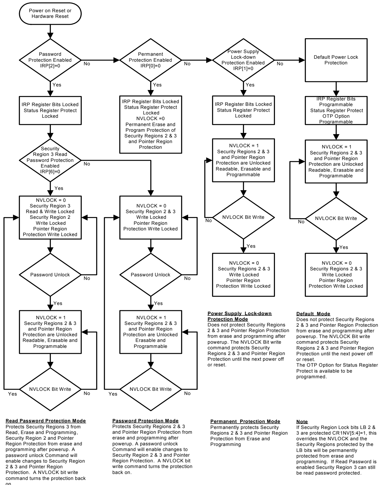
図 26. 永久的保護、パスワード保護および電源ロックダウン保護の概要
