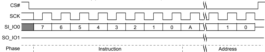
図 99. IBUL コマンド シーケンス
