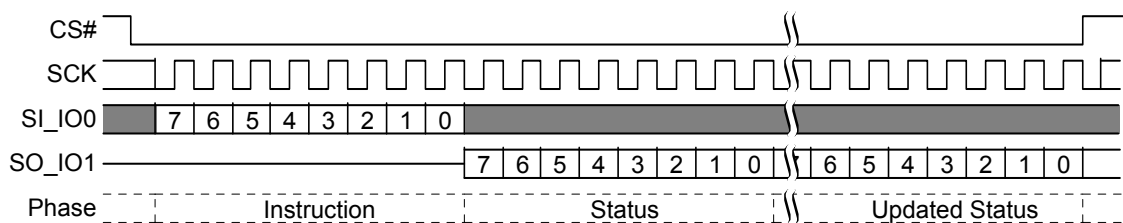
図 37. ステータス レジスタ 2 読み出し (RDSR2) コマンド
