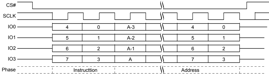
図 85. ブロック消去 (BE D8h または 4BE DCh) コマンド シーケンス – QPI モード
