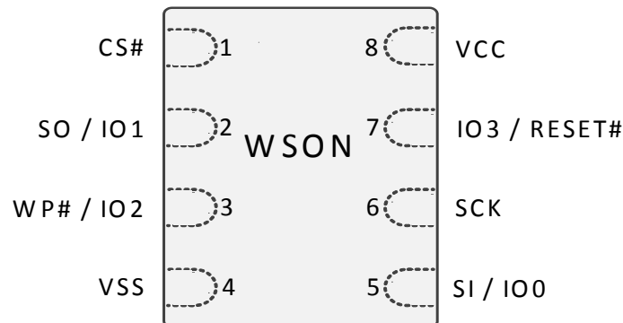
図 3. 8 コネクタ パッケージ (WSO 6x8) (WSO 5x6)、上面図
