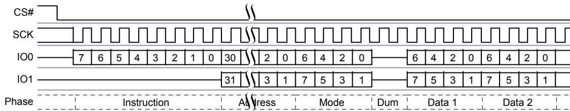
図 19. デュアル I/O コマンド
