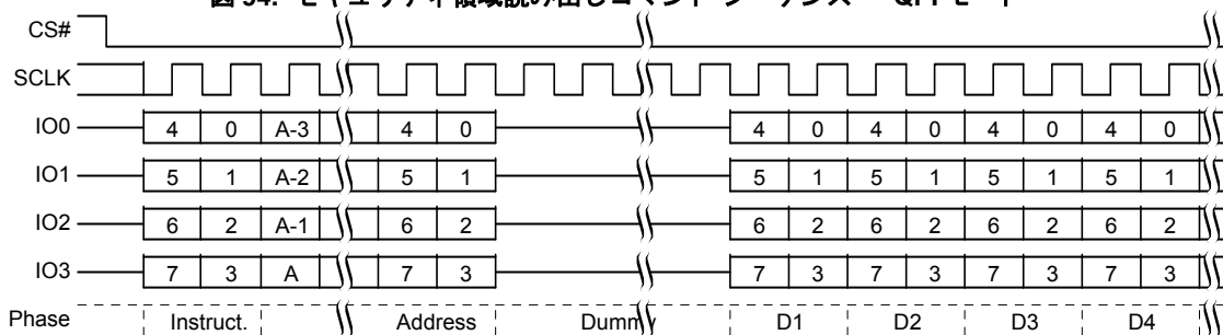
図 94. セキュリティ領域読み出しコマンド シーケンス - QPI モード
