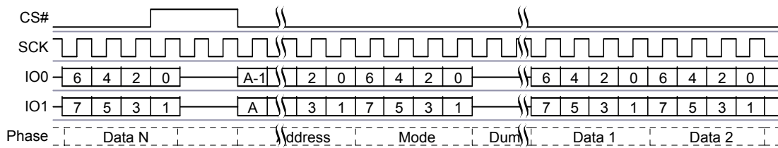
図 70. デュアル I/O 連続読み出しコマンド シーケンス
