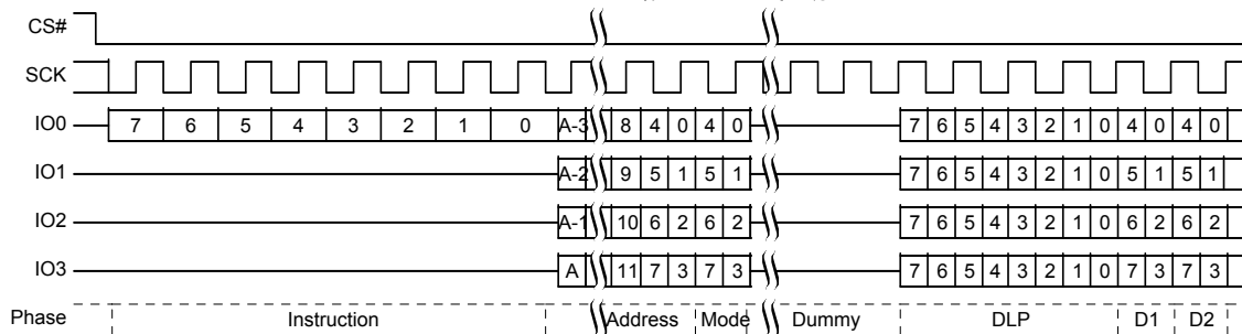
図 74. DDR クアッド I/O 読み出しの初期アクセス
