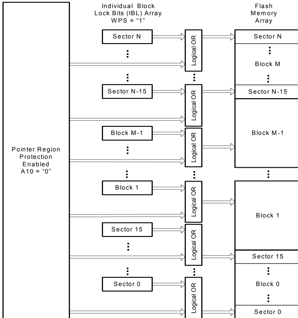
図 25. 個別ブロックロック/ポインター領域保護の制御
