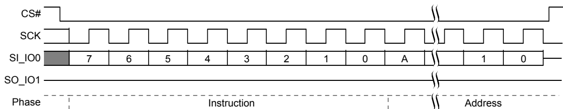
図 82. ハーフ ブロック消去 (HBE 52h または 4HBE 53h) コマンド シーケンス
