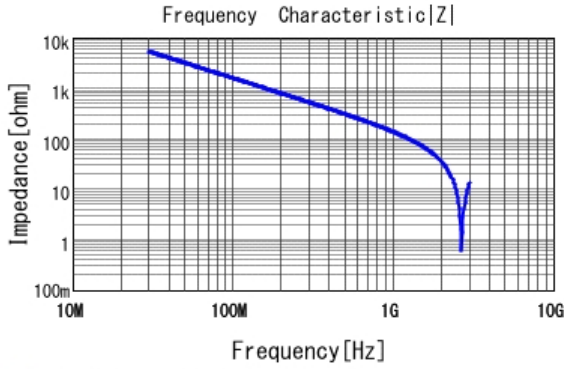
■ RCE5C1H1R0C0A2H03B |Z| DCOV, 25degC
