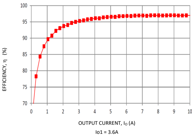
Fig 9a: Efficiency
