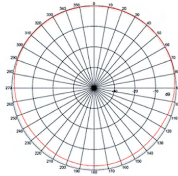
E-plane 5.5 GHz
