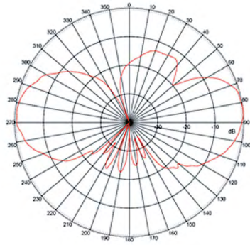
H-plane 5.5 GHz
