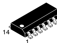
SOIC-14 NB CASE 751A-03
