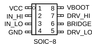
SOIC-8
