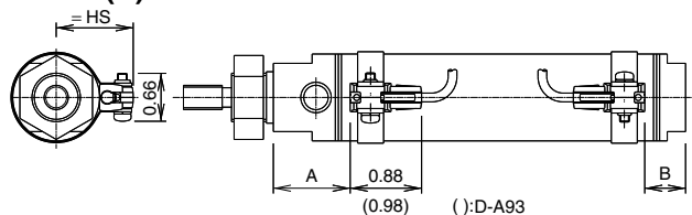
D-A9□(V)
