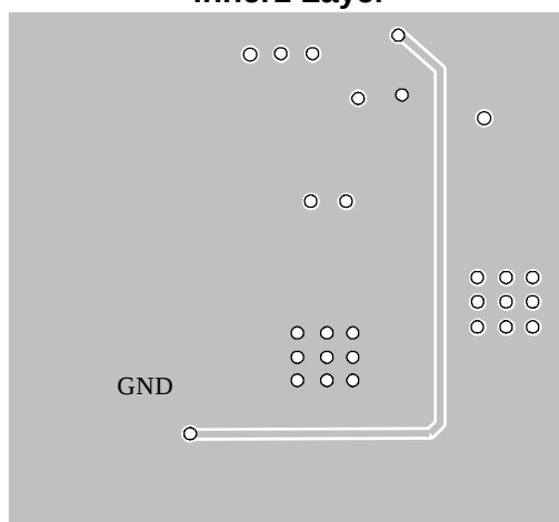
Inner2 Layer
