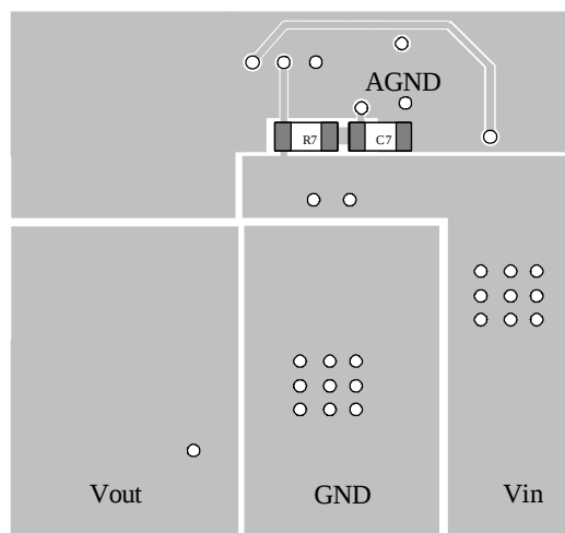
Bottom Layer
