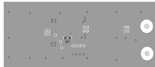
Bottom Layer
