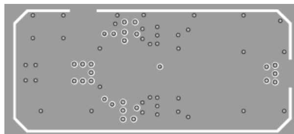
Inner Layer 1
