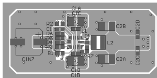
Top Layer
