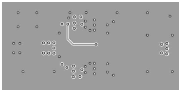
Bottom Layer
