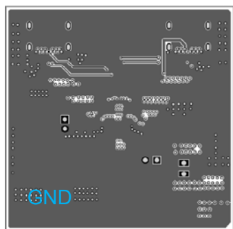
Middle Layer 2
