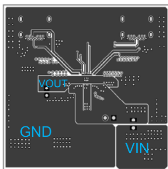
Middle Layer 1
