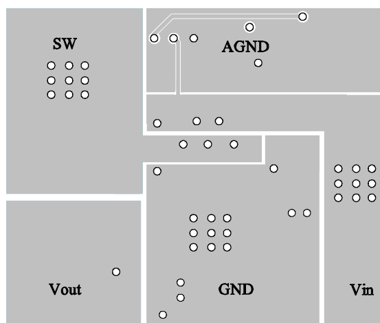
Bottom Layer
