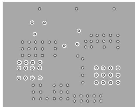
Bottom Layer
