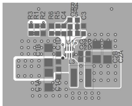
Top Layer
