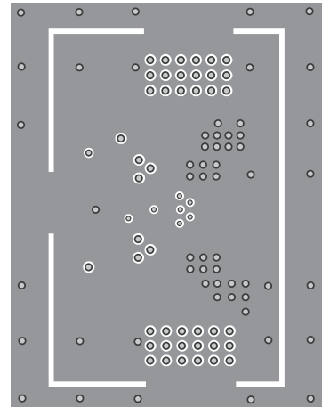
Inner Layer 1
