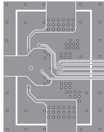
Inner Layer 2
