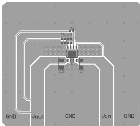
Top Layer
