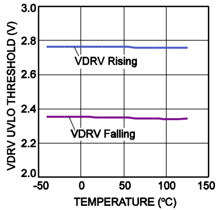
VDRV UVLO
