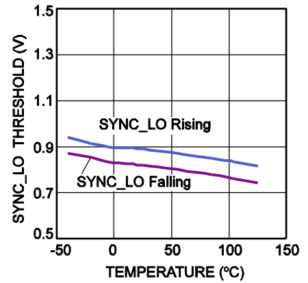
Sync_Lo
