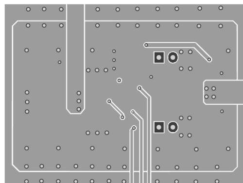
Inner Layer 2
