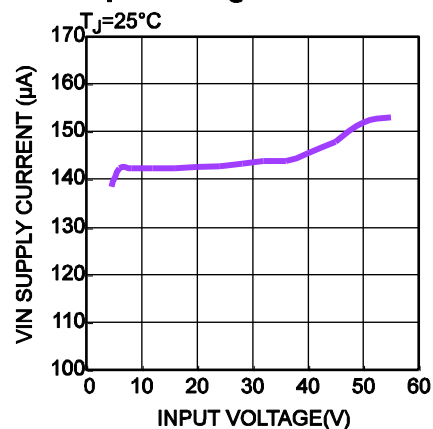
Vin Quiescent Current vs. Input Voltage
