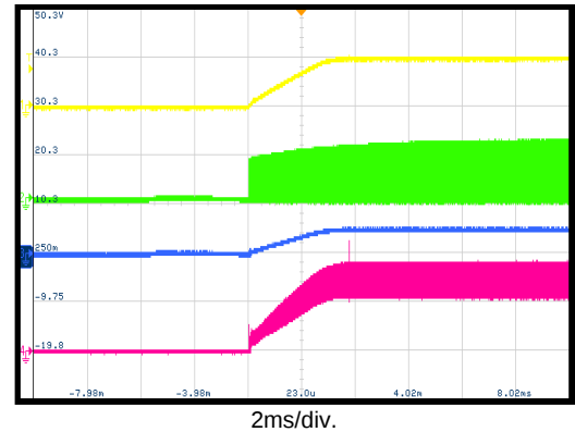
VIN Start-Up
