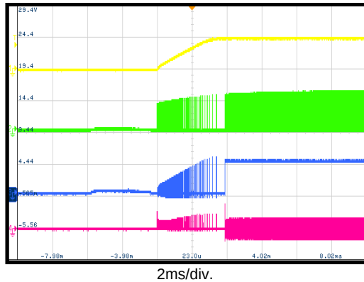
VIN Start-Up
