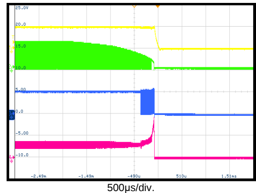
VIN Shutdown
