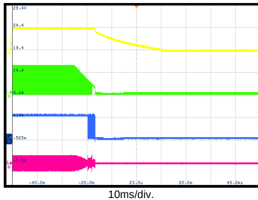
VIN Shutdown
