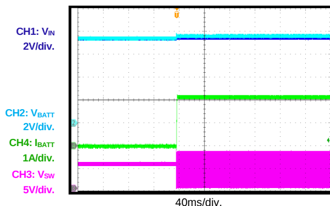
Boost Enabled
