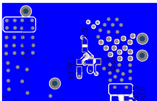
Bottom Layer
