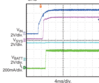
En Off, Charge Mode
