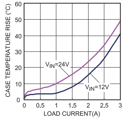
Thermal Rise
