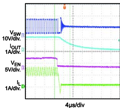
EN Shutdown
