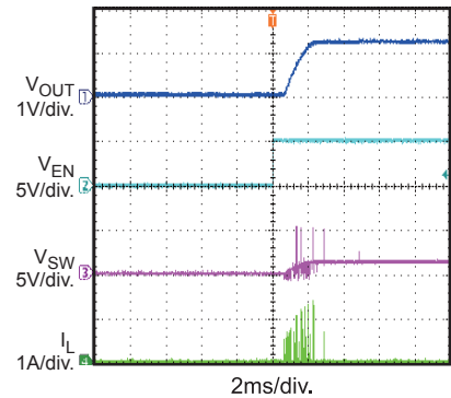
Enable On
