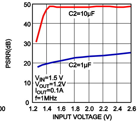
PSRR vs. VIN
