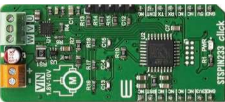
STSPIN233 Click
