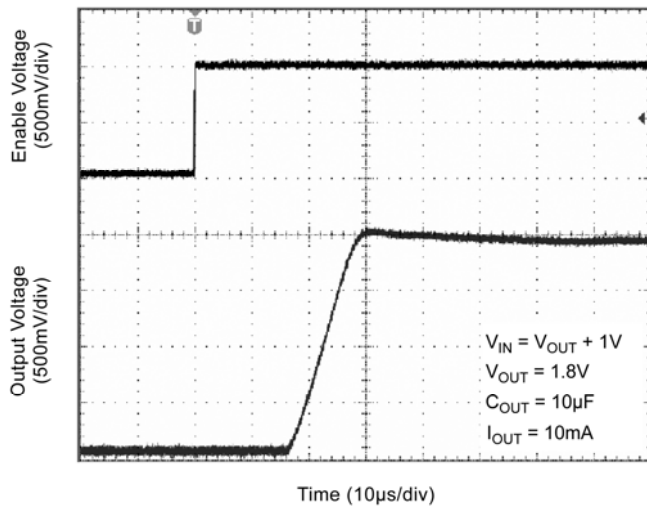
Enable Turn-On
