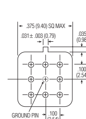
MGA/MGAD/MGADD HEADER
