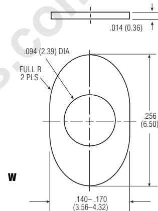
MGAT MOUNTING PAD
