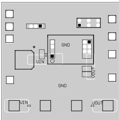
Top Layer
