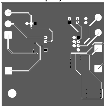
Mid Layer 2
