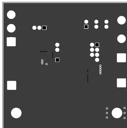
Mid Layer 1
