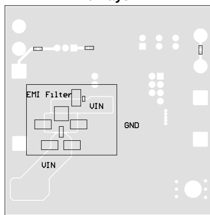
Bottom Layer
