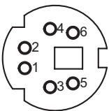
MD-90J
